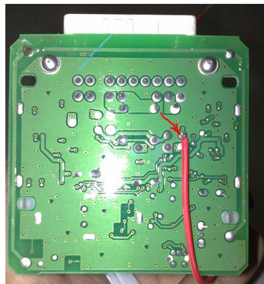
Рис. 1 Блок центрального замка
